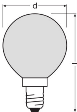
SPC.P OVEN FR 40 W 240 V E14
