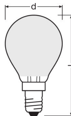
BASE CLAS P 40 FR 4 W/2700K E14
